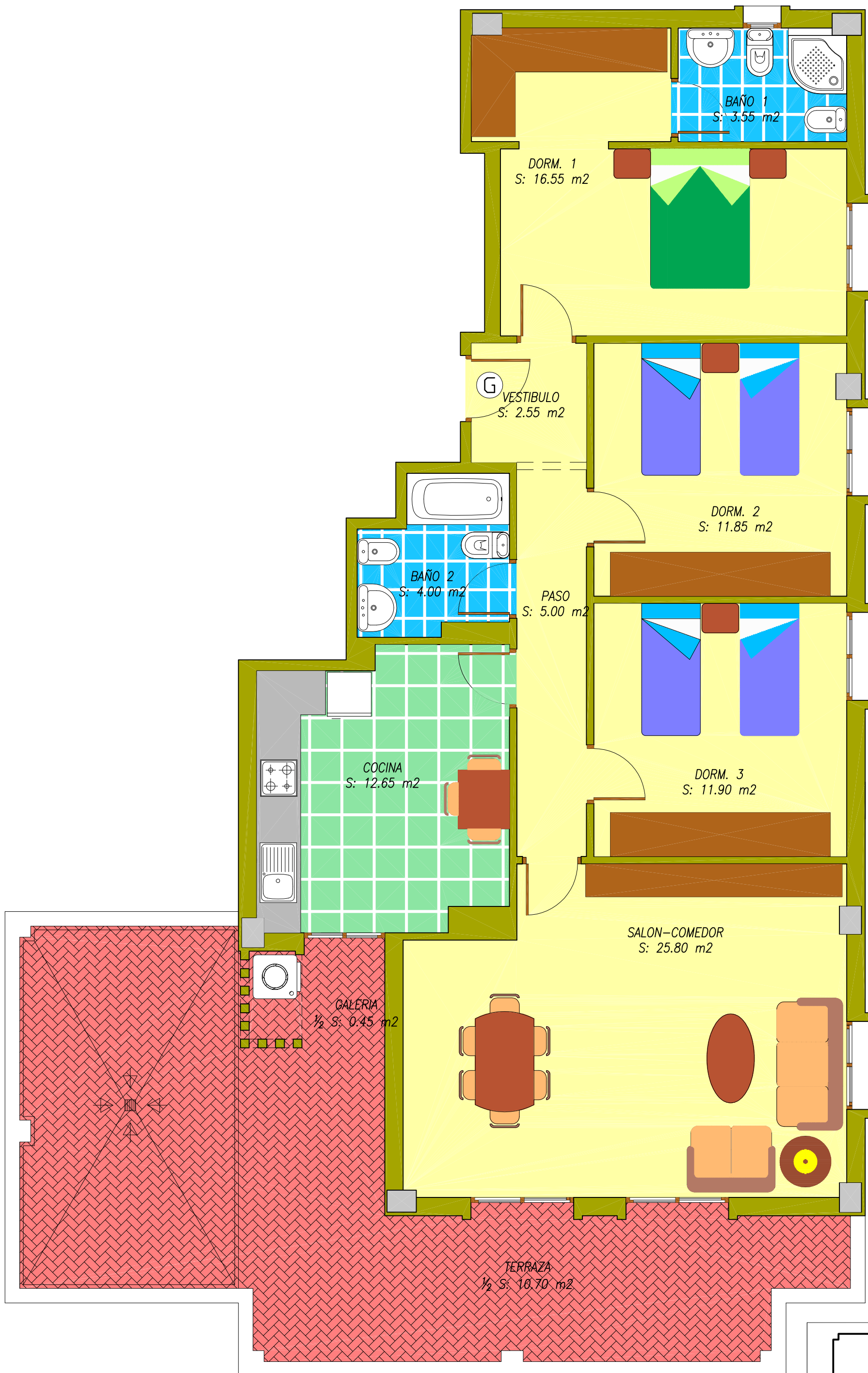
VIVIENDA TIPO G PLANTA PISO 5°
